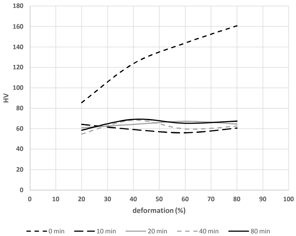
CuAs-10: HV vs. deformation (%)
