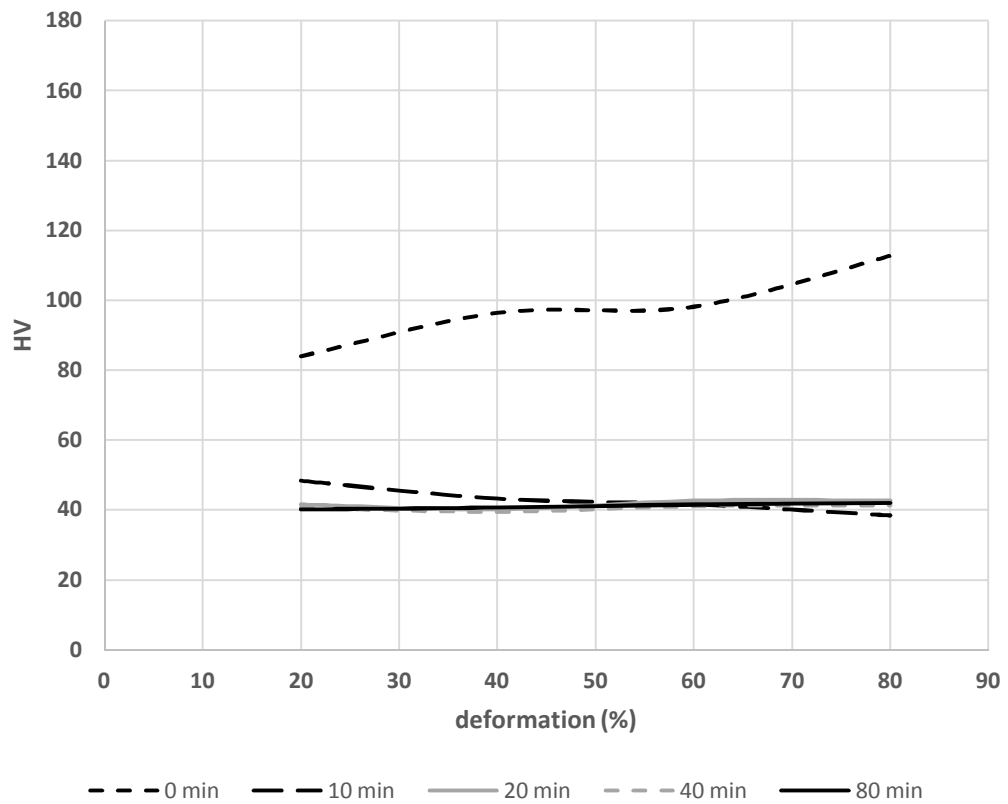
CuAs-4: HV vs. deformation (%)
