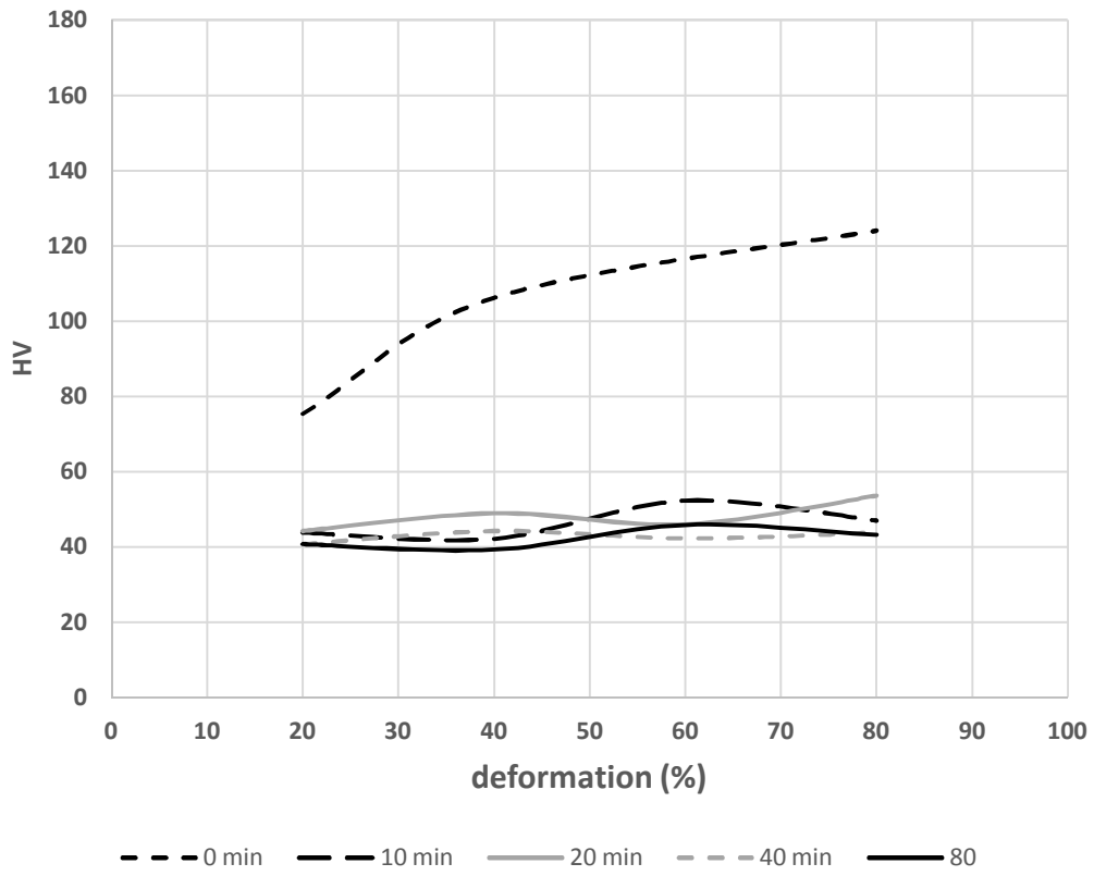
CuAs-5: HV vs. deformation (%)
