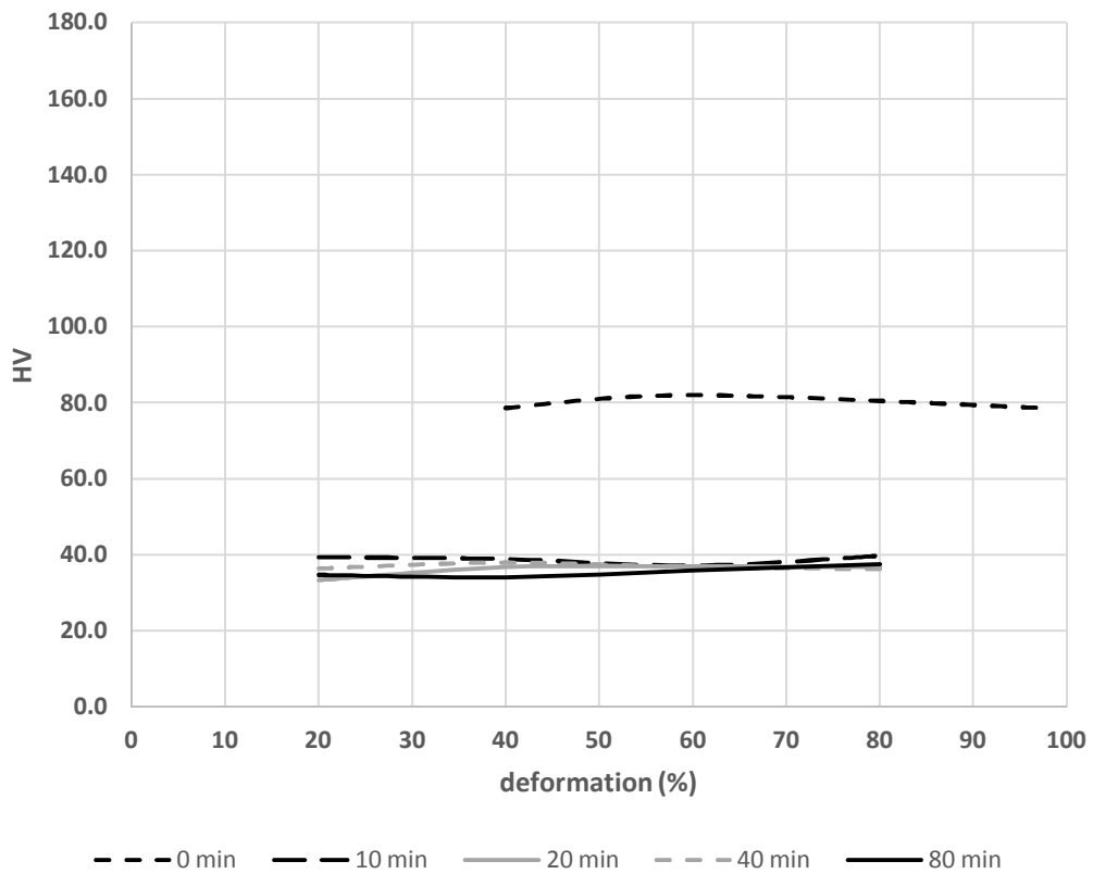
CuAs-2: HV vs. deformation (%)
